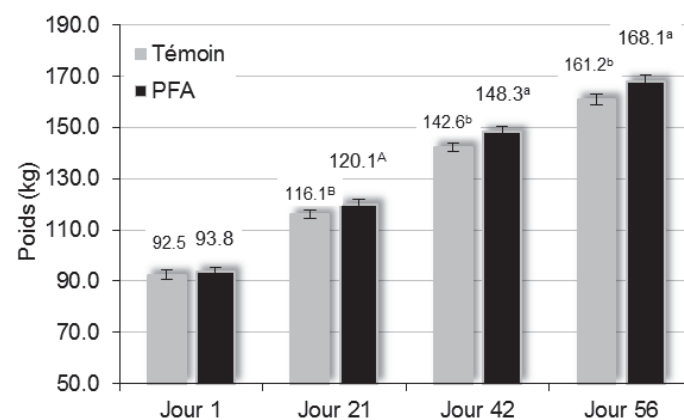
Figure 1 : Effets d'une supplémentation de l'AA et du CS en PFA sur l'évolution du poids. a,b Différence significative entre les groupes (p < 0,05); A,B tendance se rapprochant d'une différence significative (p < 0,10)
